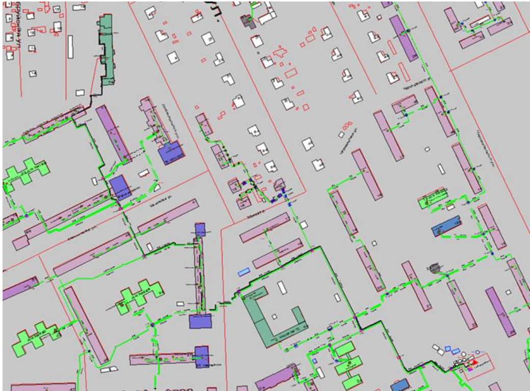
Рисунок 3.43 – Трассировка теплопровода от котельной АО «Теплоэнерго» по ул. Баранова, д. 11 до конечного потребителя «ПТ-Мечн, 74 маст»
