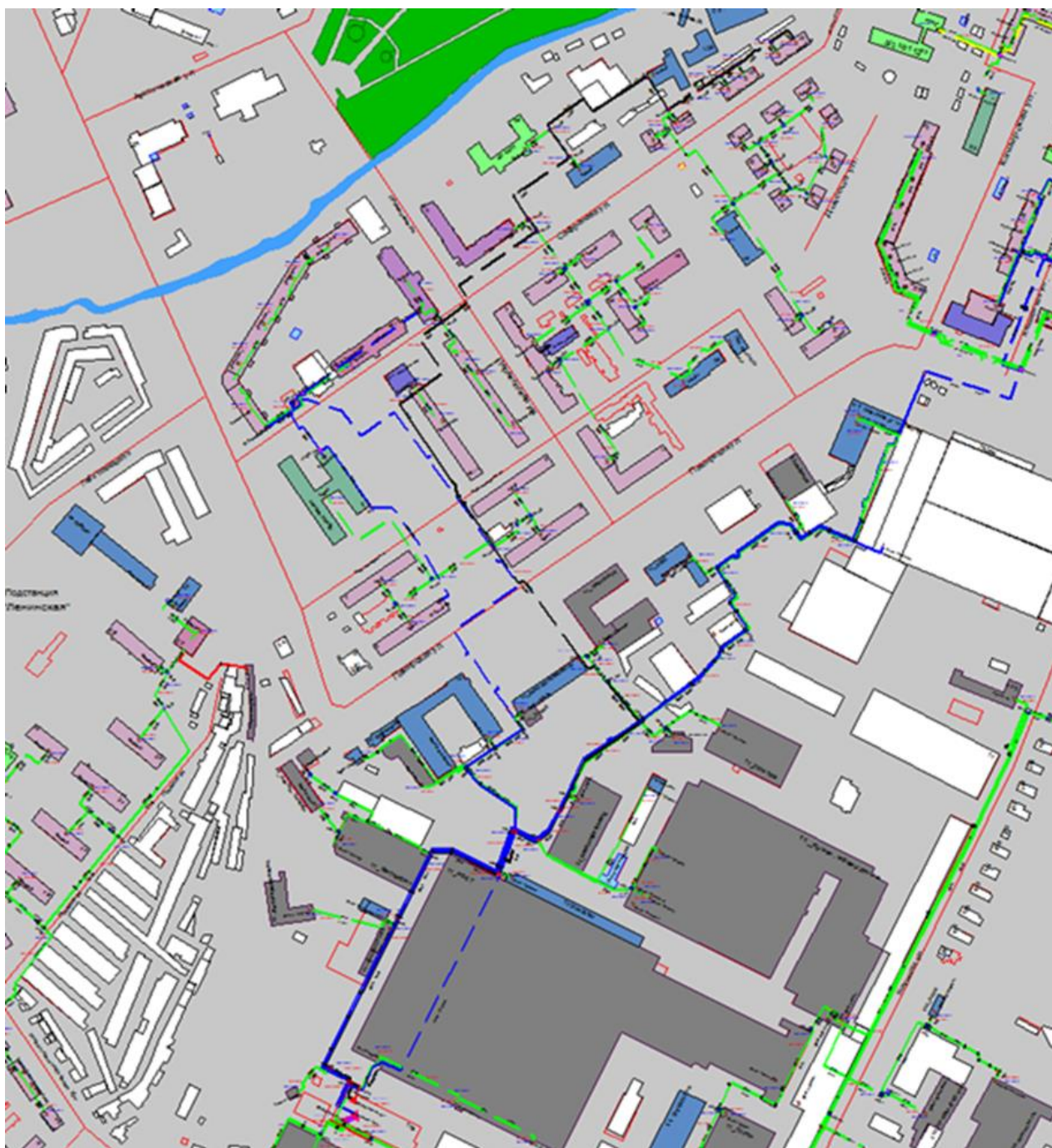
Рисунок 3.31 – Трассировка теплопровода от котельной АО «Теплоэнерго» по ул. Памирская, д. 11 до конечного потребителя «ПТ-Сафрон,15 вв2»
